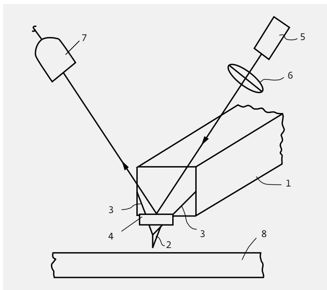
Рис.1. Современная схема АСМ: 1 – держатель; 2 – зонд, игла; 3 – гибкая консоль; 4 – зеркало; 5 – лазер; 6 – объектив; 7 – фотоприемник; 8 – поверхность образца
