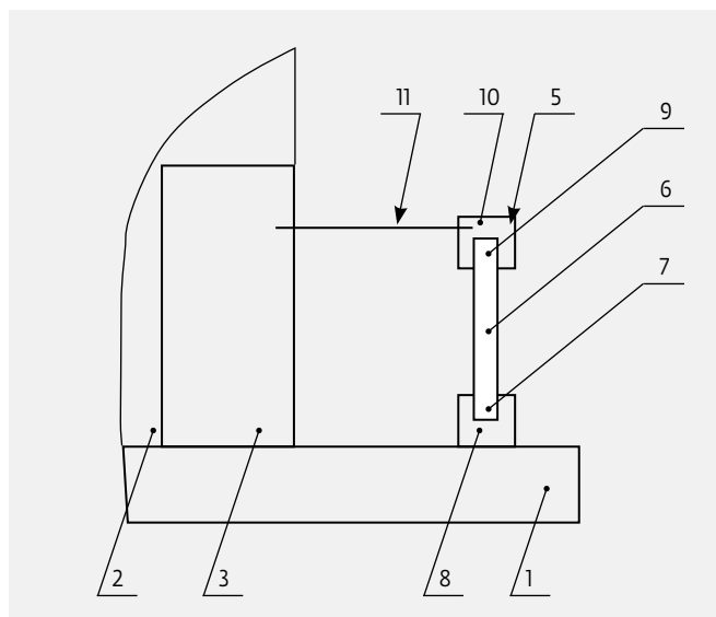
Рис.3. Вариант выполнения привода для перемещения в нанометровом диапазоне 1 - основание, 2 - блок, 3 - модуль, 5 - привод, 6 - пьезобиморф, 7 - первый конец пьезобиморфа, 8 - первый держатель 9 - второй конец пьезобиморфа, 10 - второй держатель, 11 - упругий элемент
